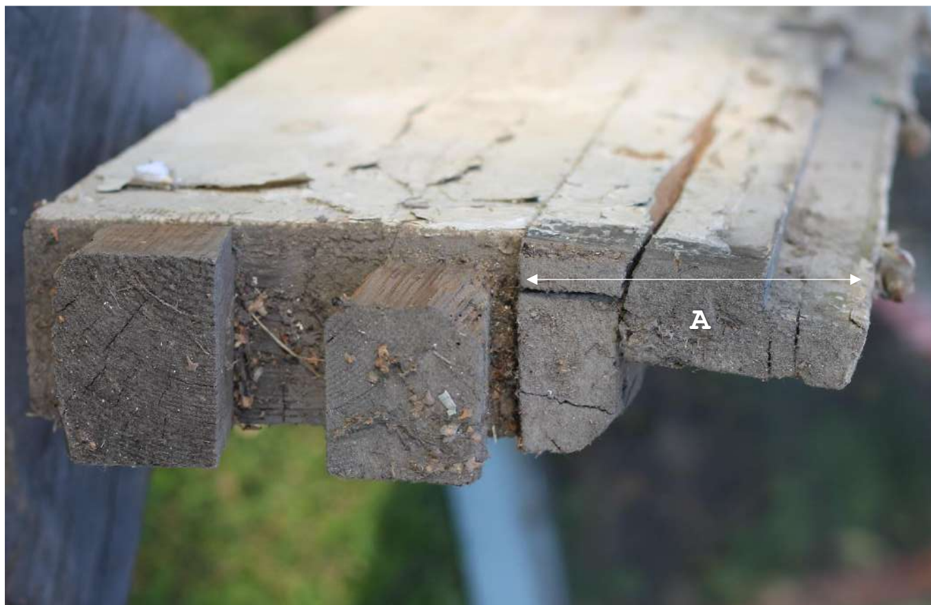
55.fotoattēls. Sākotnējā loga aploda, kas pagarināta (A) 19.gs. beigās, kad fasādes apšuj ar dēļiem.
