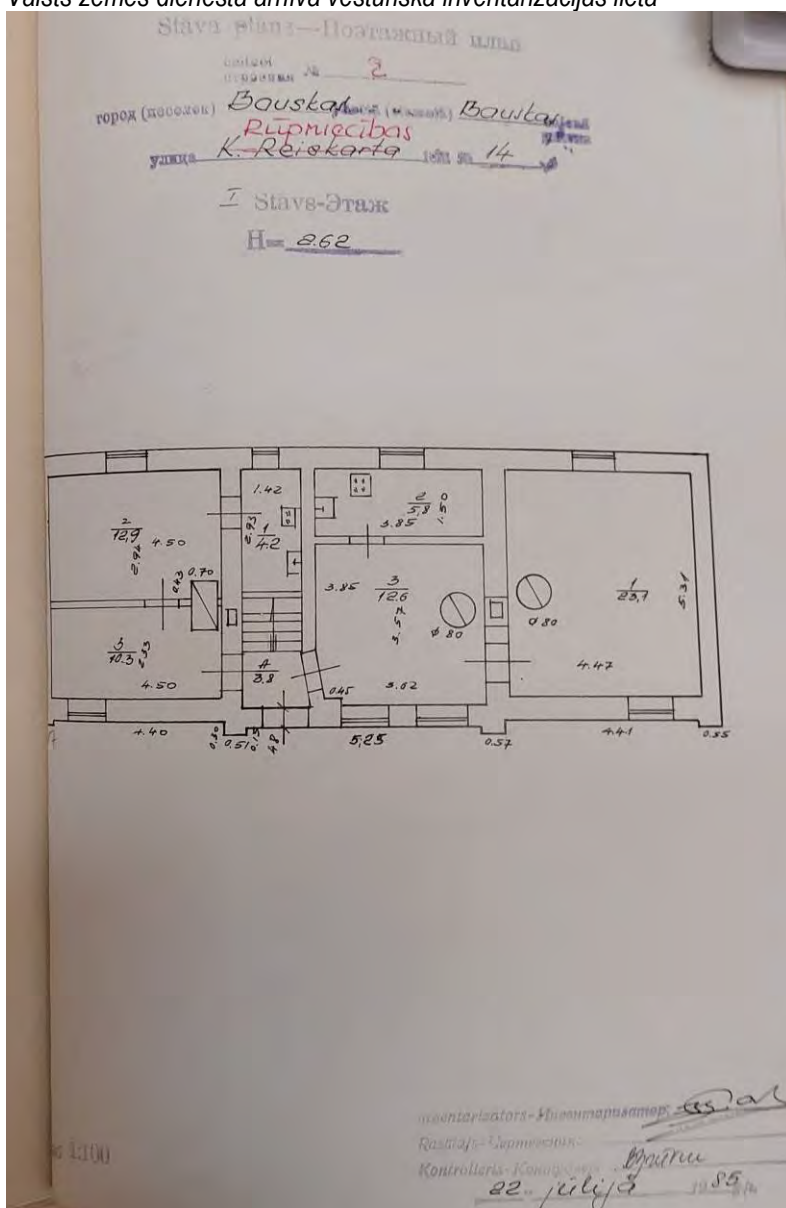
1985.g. Pagalma ēka. Pirmā stāva plāns.
