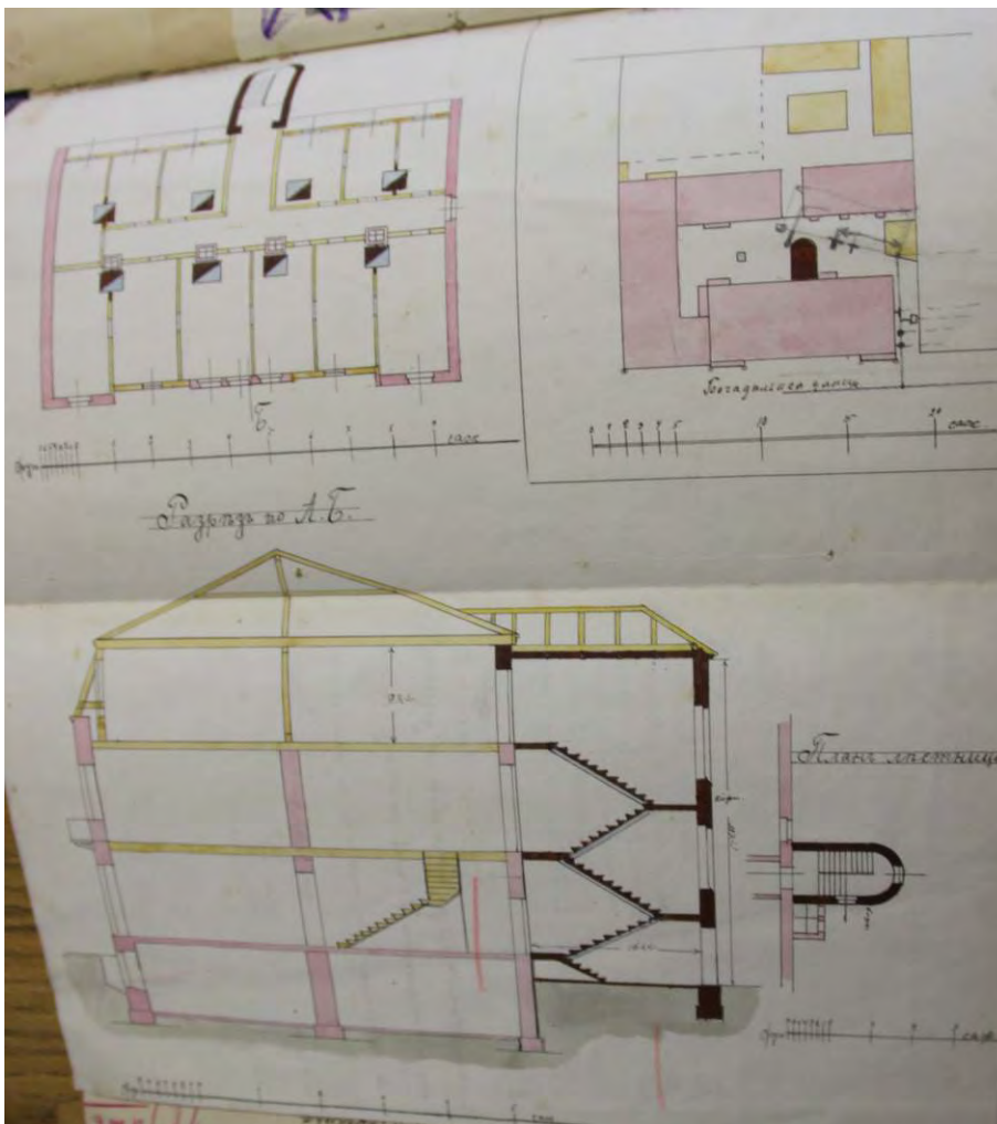
1912.g. Ielas ēka. Kāpņu telpas piebūves projekts.
