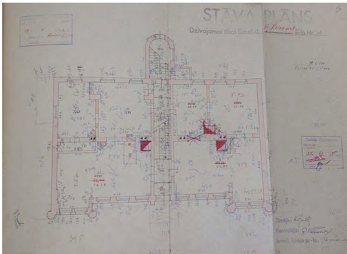
1948.g. ielas ēka. Pirmā stāva plāns.
