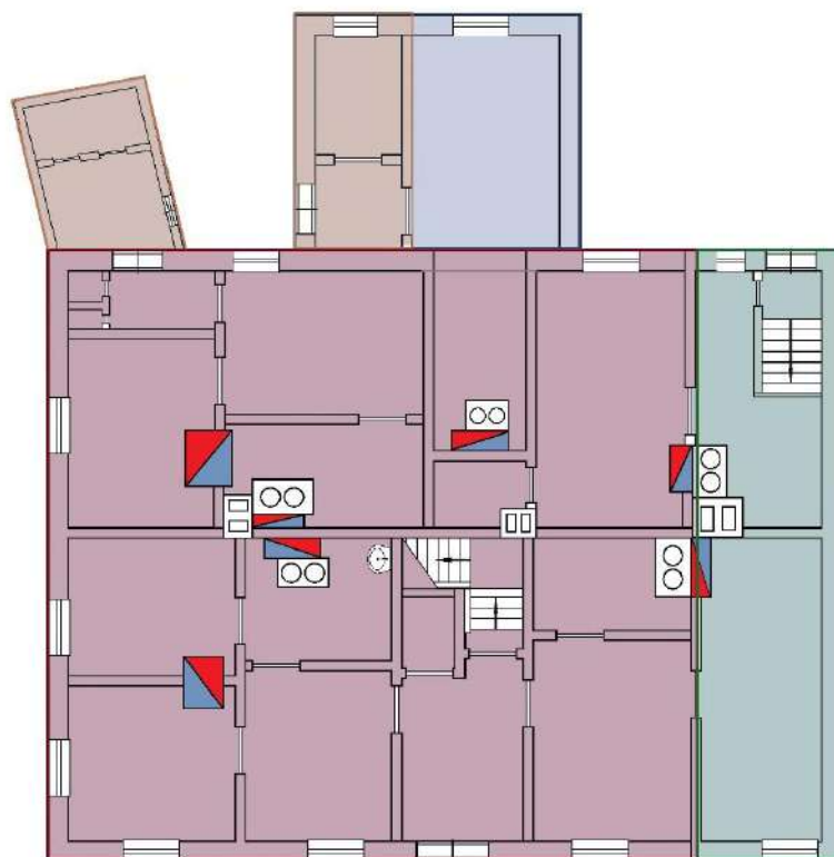
60. attēls. Ēkas 1. stāva plāns ar shematiski marķētiem dažādu būvperiodu apjomiem.
