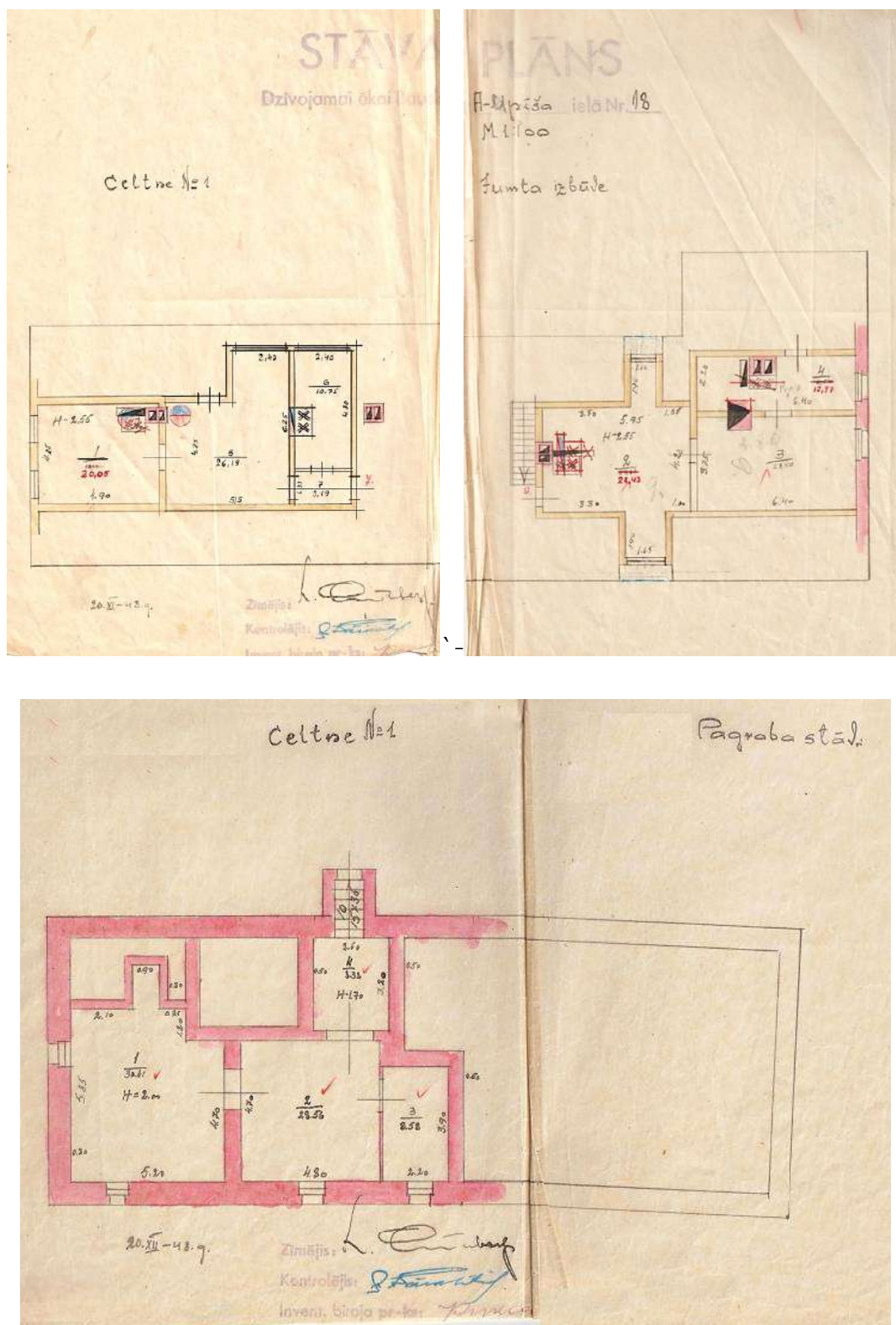
32., 33. attēls. Ēkas pagraba un bēniņu stāva plāni. Ēkas inventarizācijas lieta, 1948. gads. Lieta glabājas pie mājas vecākā.
